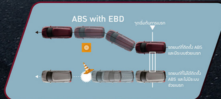
ระบบป้องกันล้อล็อก (ABS) ช่วยป้องกันล้อล็อกขณะเบรกกะทันหัน พร้อมเพิ่มประสิทธิภาพในการหักหลบสิ่งกีดขวาง เพื่อความปลอดภัยสูงสุด ระบบกระจายแรงเบรก (EBD) เทคโนโลยีที่ช่วยกระจายแรงเบรกให้ทุกล้อ เบรกได้อย่างสมดุลในระนาบที่สั่นไหว ควบคุมการขับขี่ได้ทุกสถานการณ์
